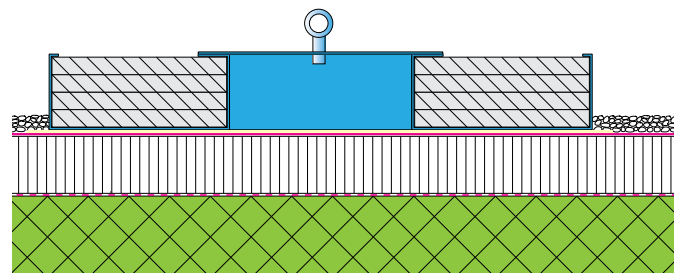
Abb. 4: Ausstattungsstufe 1: Anschlagpunkte mit Auflast ohne Durchdringungen der Abdichtung. Diese Punkte können temporär eingesetzt werden, dürfen jedoch bei frostigen Temperaturen für Arbeiten, wie z. B. Schnee räumen, nicht verwendet werden.
