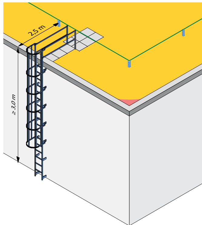
Abb. 20: Zugang über eine fix montierte Leiter
