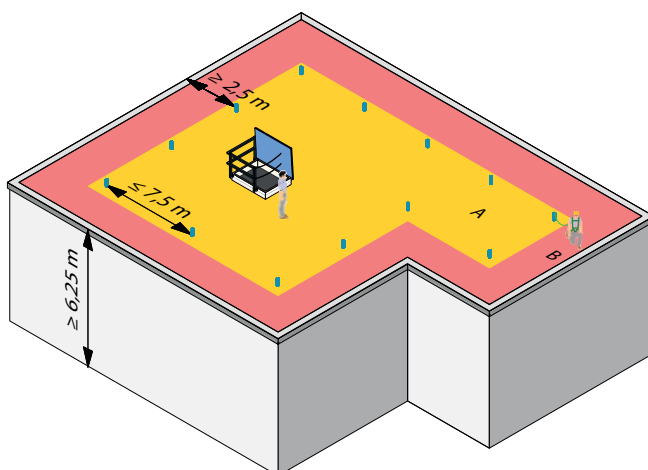
Abb. 2: Ausstattungsstufe 1: EAP am Dachrand entlang der Geometrie des Gebäudes angepasst
