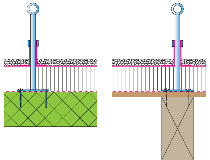
Abb. 3: Ausstattungsstufe 1: EAP auf einem wärmegegliederten Flachdach eingebaut, Variante auf einer Beton- und einer Holzunterkonstruktion
