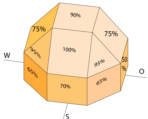
Wirkungsgrad der Ausrichtungsflächen am Gebäude
